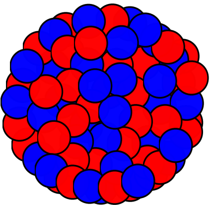
Uranium 238
