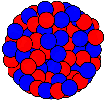
Uranium 238
