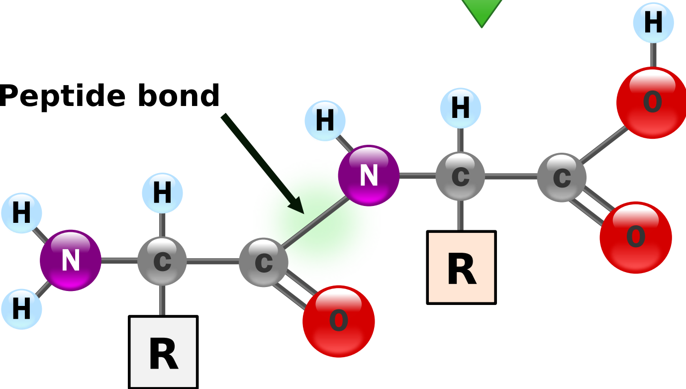
Dipeptide
