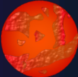
Venus
