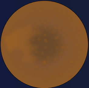
Mercurio
