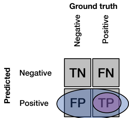
Precision
